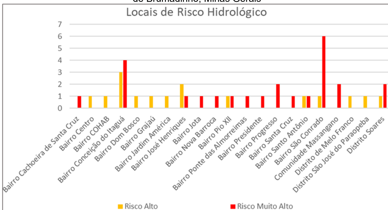
Figura 04 – Distribuição de risco hidrológico, por locais visitados em 2022, no Município de Brumadinho, Minas Gerais
