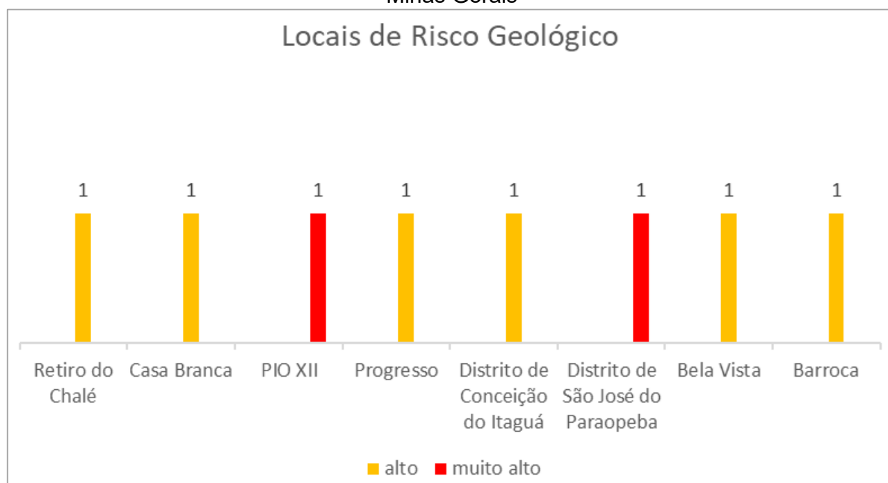
Figura 02 – Locais de risco geológico visitados em 2022, Município de Brumadinho, Minas Gerais
