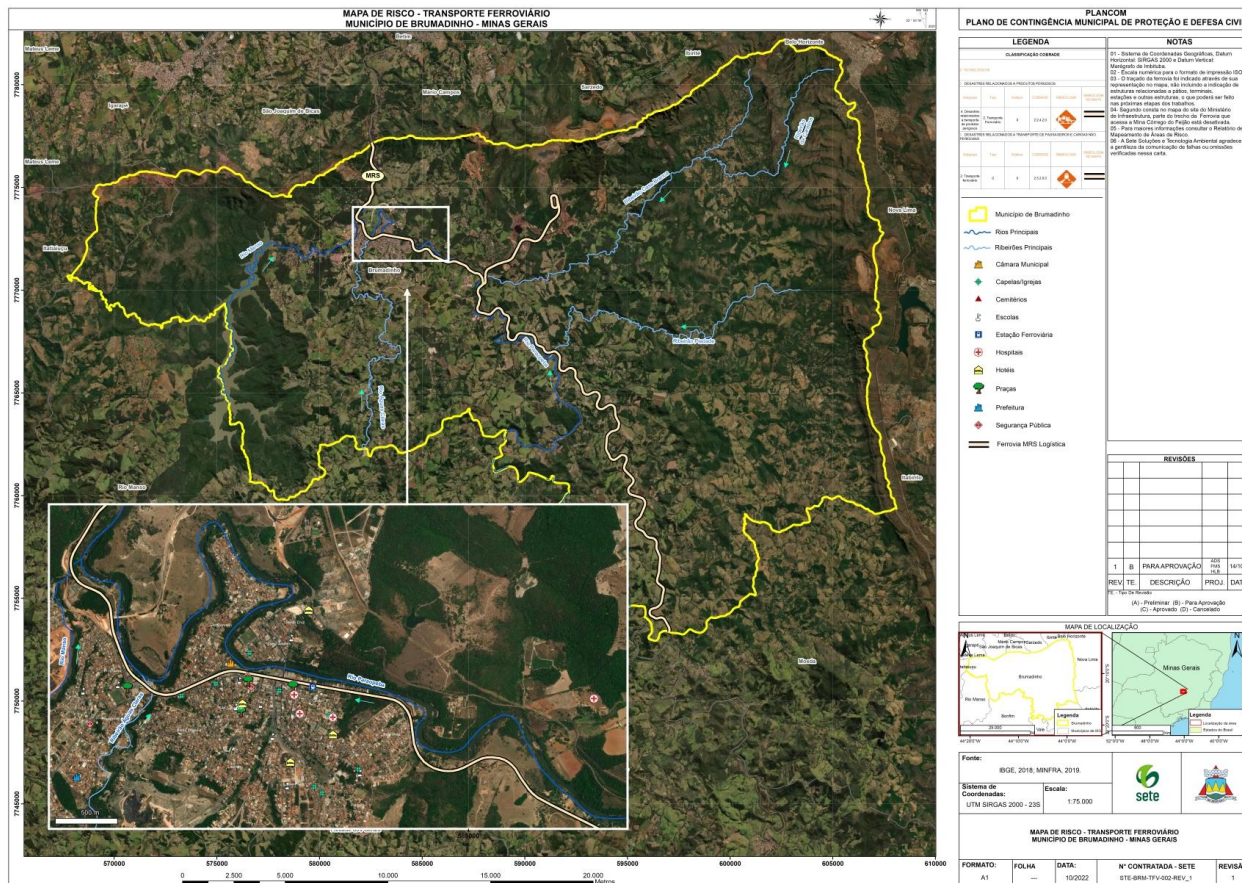
Figura 06 – Mapa de setorização de risco tecnológico de transporte ferroviário de Brumadinho, Minas Gerais
