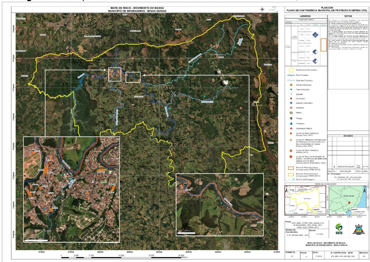
Figura 01 – Mapa de risco a movimentos de massa de Brumadinho, Minas Gerais
